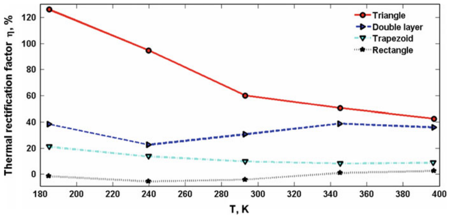
Fig. 3 Thermal rectification factor
